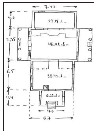
План деревянной Троицкой церкви 1931 год
