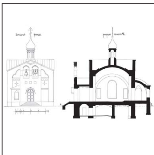
Проект непостроенного каменного храма 1912 год
