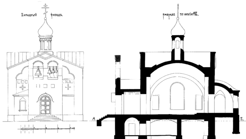
Проект непостроенного каменного Троицкого храма. 1912 год. Из фондов ЦГАМ.
