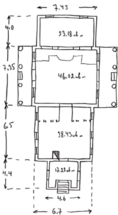
План деревянной Троицкой церкви. 1931 год. Из фондов ЦГАМО.
