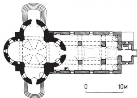
Общий вид и план Покровского храма
